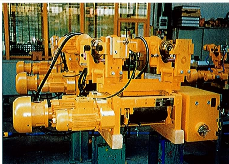
Paranchi elettrici a fune in esecuzione speciale Wire rope electric hoists in special execution
